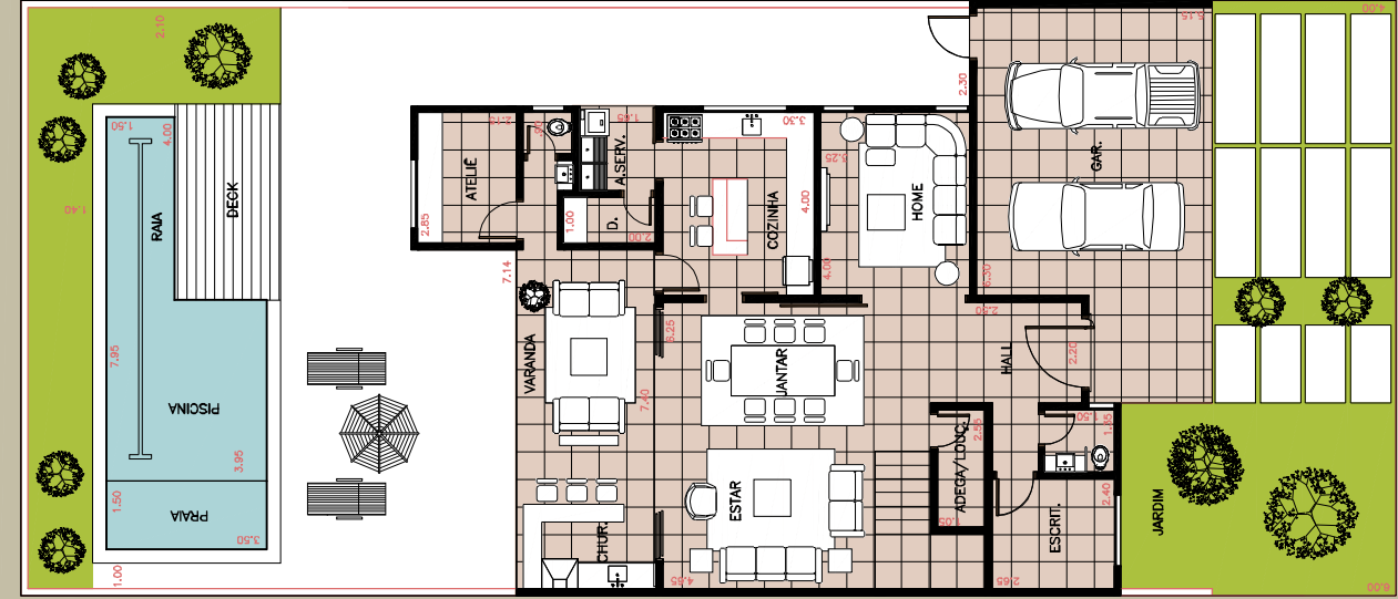
PLANTA TÉRREA
