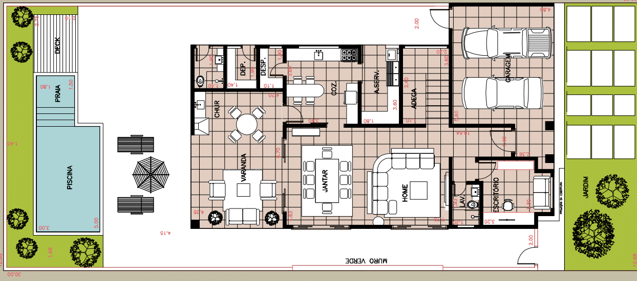
PLANTA TÉRREA
