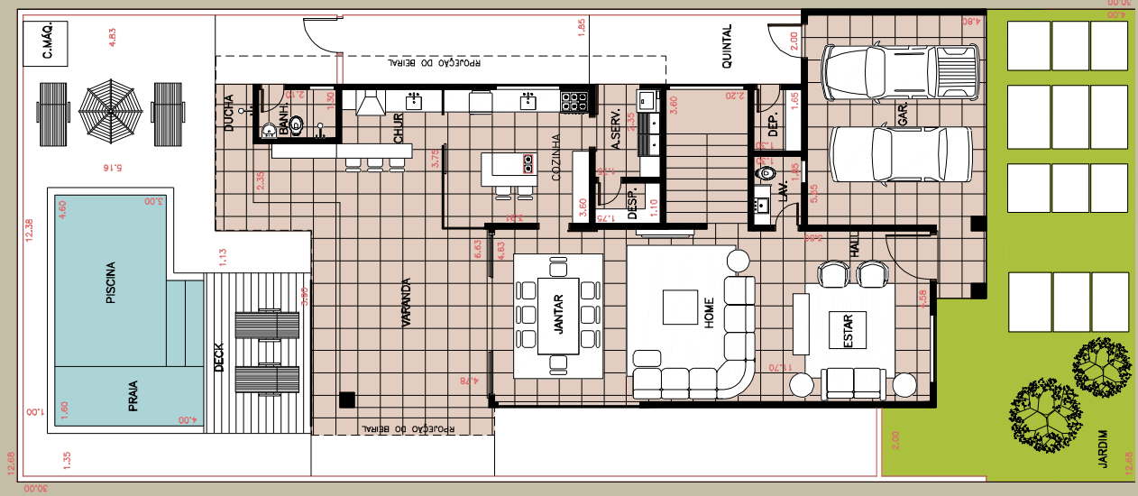
PLANTA TÉRREA
