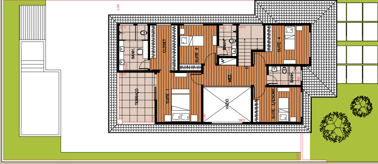
PLANTA SUPERIOR
