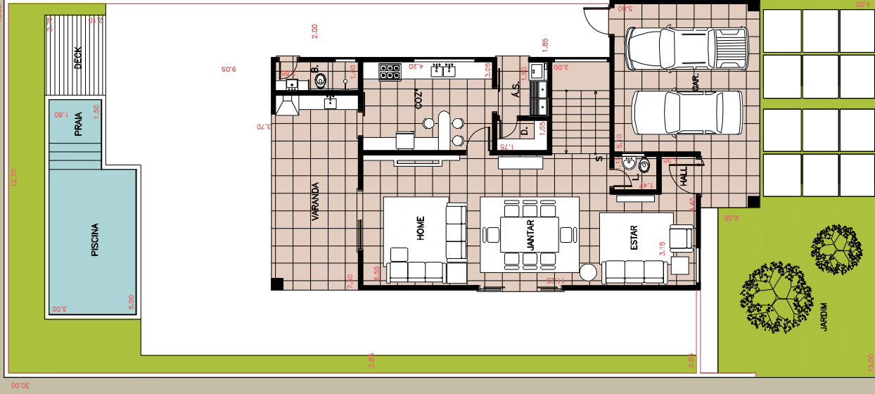
PLANTA TÉRREA
