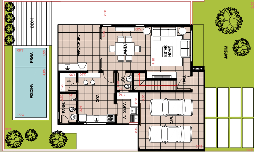
PLANTA TÉRREA
